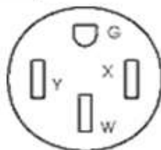
Nema 14-50
